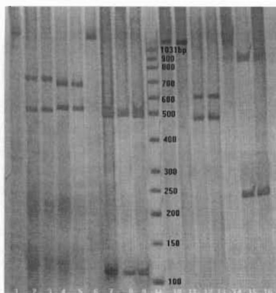
شکل ۱: الکتروفورز محصول PCR هضم شده توسط آنزیم HinfI با ژل پلی آکریل آمید ۶ درصد، ستون آنزیم PCR ماهی سس، ستون ۲-۳ ماهی سس، ستون ۴-۵ ماهی سیم، ستون ۶ PCR ماهی سیم، ستون ۷-۹ ماهی کلمه، ستون ۱۰ PCR ماهی کلمه، ستون ۱۱ PCR ماهی سیم
