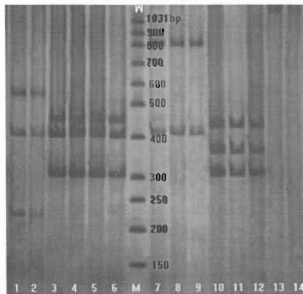
شکل ۴: الکتروفورز محصول PCR هضم شده توسط آنزیم RsaI با ژل پلی آکریل آمید ۶ درصد، ستون ۱-۲ ماهی سس، ستون ۳-۶ ماهی کلمه، ستون ۷-۹ ماهی سیم، ستون ۱۰-۱۲ ماهی ماش، ستون ۱۳-۱۴ ماهی سفید، ستون M مارکر
