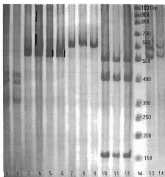
شکل ۲: الکتروفورز محصول PCR هضم شده توسط آنزیم HhaI با ژل پلی آکریل آمید ۶ درصد، ستون ۱-۲ ماهی سس، ستون ۳-۶ ماهی کلمه، ستون ۷-۹ ماهی سیم، ستون ۱۰-۱۲ ماهی ماش، ستون ۱۳-۱۴ ماهی سفید، ستون M مارکر
