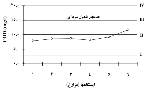
شکل ۳: تغییرات اکسیژن محلول، درصد اشباعیت، اکسیژن خواهی بیولوژیک و شیمیایی در ایستگاه‌ها (مزارع پرورش ماهی قزل آلا) به‌همراه حد مجاز در رودخانه هراز (سال ۹۷-۱۳۹۶)
