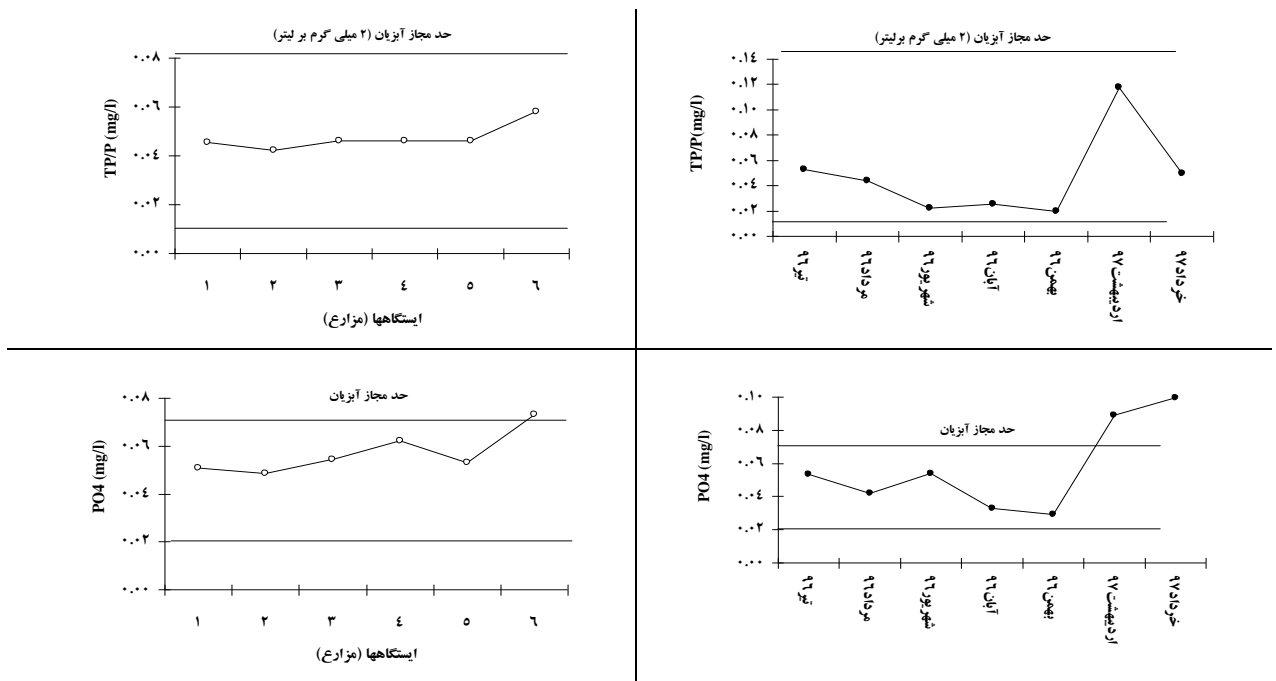
شکل ۵: تغییرات فسفرکل و فسفات در ماهها و ایستگاهها (مزارع پرورش ماهی قزل آلا) به همراه حد مجاز در رودخانه هراز (سال ۹۷-۱۳۹۶)
