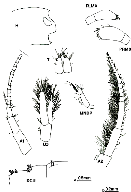
شکل ۳: مقیاس‌ها: (PLMX و PRMX) b، (MNDP، DCU، A2، A1، T و H) a: سر، T: تلسون، A1: شاخک ۱، A2: شاخک ۲، DCU: شاخک ۱، U3: ناحیه پشتی بندهای دم، U: پای دم، MNDP: پای دم، PRMX: پالپ آرواره فوقانی، PLMX: پالپ آرواره تحتانی راست، PLMX: پالپ آرواره تحتانی چپ
