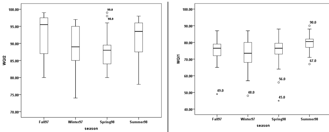
شکل ۴: نمودار جعبه‌ای تغییرات فصلی شاخص کیفیت آب حوزه جنوبی دریای خزر (۱۳۹۷-۹۸) (WQI1): پارامترها و وزن‌ها بر اساس مطالعات گذشته نگر (Retrospective studies) دریای خزر: پارامترها و وزن‌ها بر اساس مطالعه Nguyen و همکاران (۲۰۱۳)
