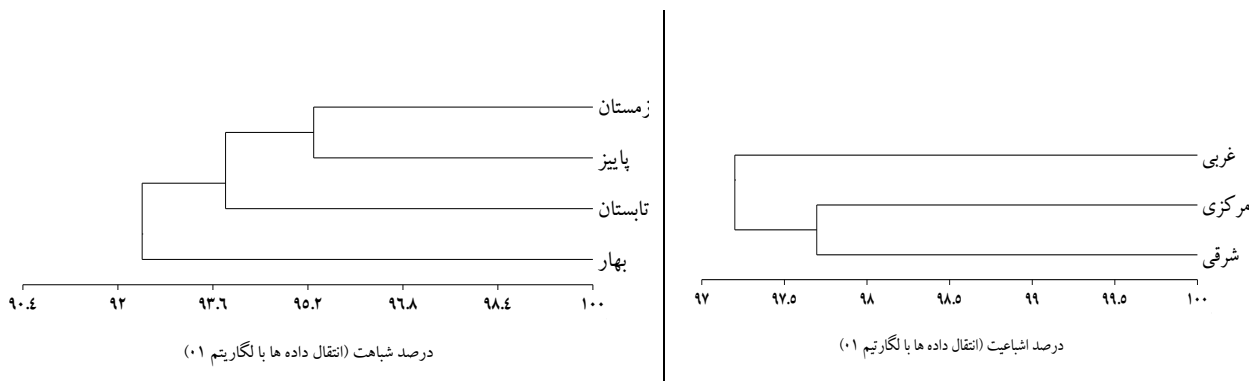
شکل ۲: نمودار خوشه‌ای بین پارامترهای شاخص کیفیت آب در فصول و مناطق مختلف حوزه جنوبی دریای خزر (۹۸-۱۳۹۷) Figure 2: Cluster diagram between water quality index parameters at different seasons and regions in the southern Caspian Sea basin (2018-2019)
