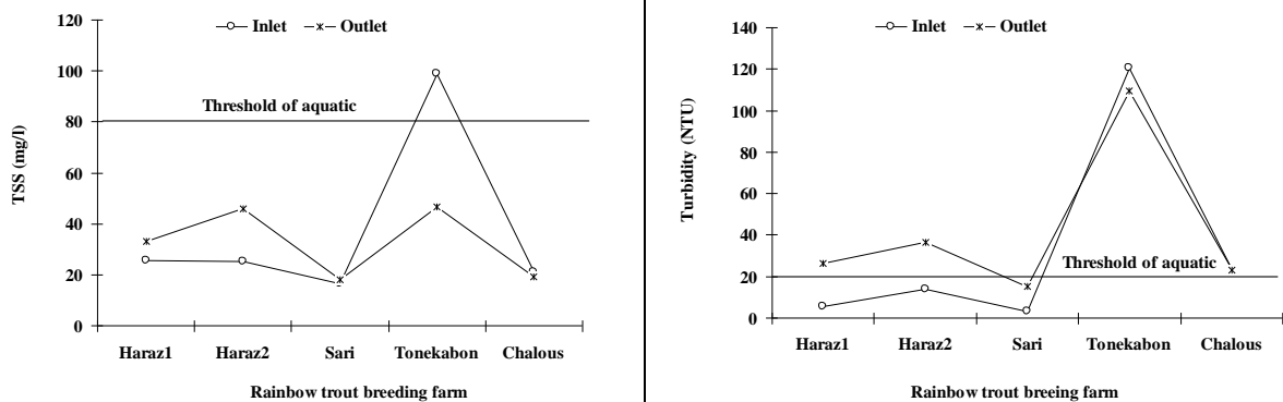
شکل ۷: تغییرات میانگین کل مواد جامد معلق و کدورت آب (NTU) در ایستگاه‌های ورودی و خروجی به همراه حد مجاز استاندارد کارگاه‌های پرورش ماهی قزل آلا منتخب استان مازندران (سال ۱۴۰۰-۱۴۰۱)
